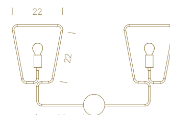
Parete doppia Double wall light
